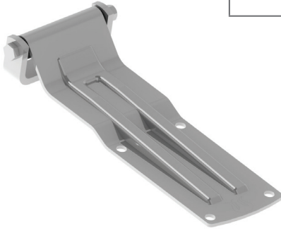
Menteşe Süper Lama Ayaklı Hinge 320/4 mm U Bracket
