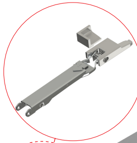
1 1010015 Dikey Kilitleme Sistemi Alüminyum Mekanizması Long Range Fastener Mechanism (Aluminium)
