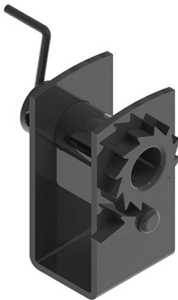
Halat Gergi Mekanizması Strap Winch (Vertical)
